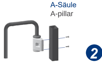
Montage von Innenseite Fahrzeug verschraubt Mounting directly bolted from vehicle side
