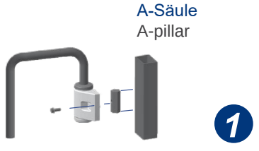
Montage von Außenseite Fahrzeug verschweißt Mounting base bolted through hex attachment
